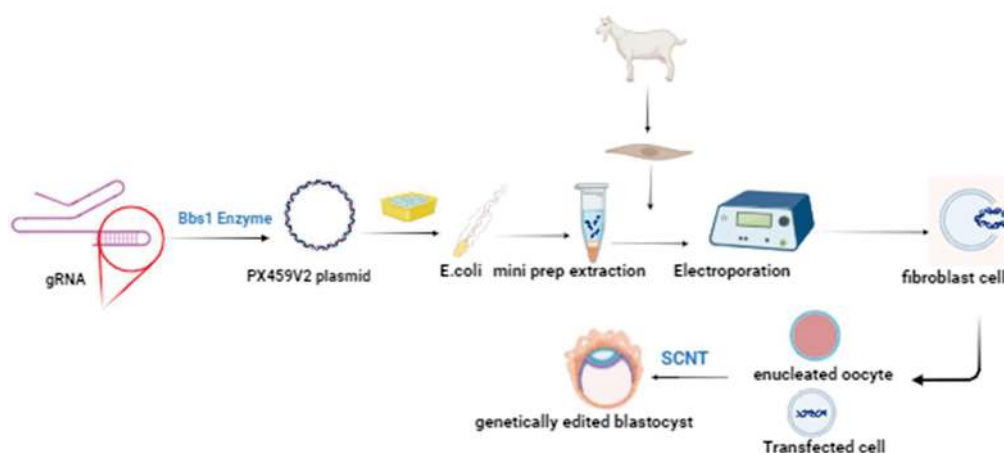
Fig. 1. Schematic diagram of different stages of DAZL gene editing in Bakhtiari goat embryo شکل ۱- شمای کلی از مراحل مختلف ویرایش ژن DAZL در رویان بز بختیاری
